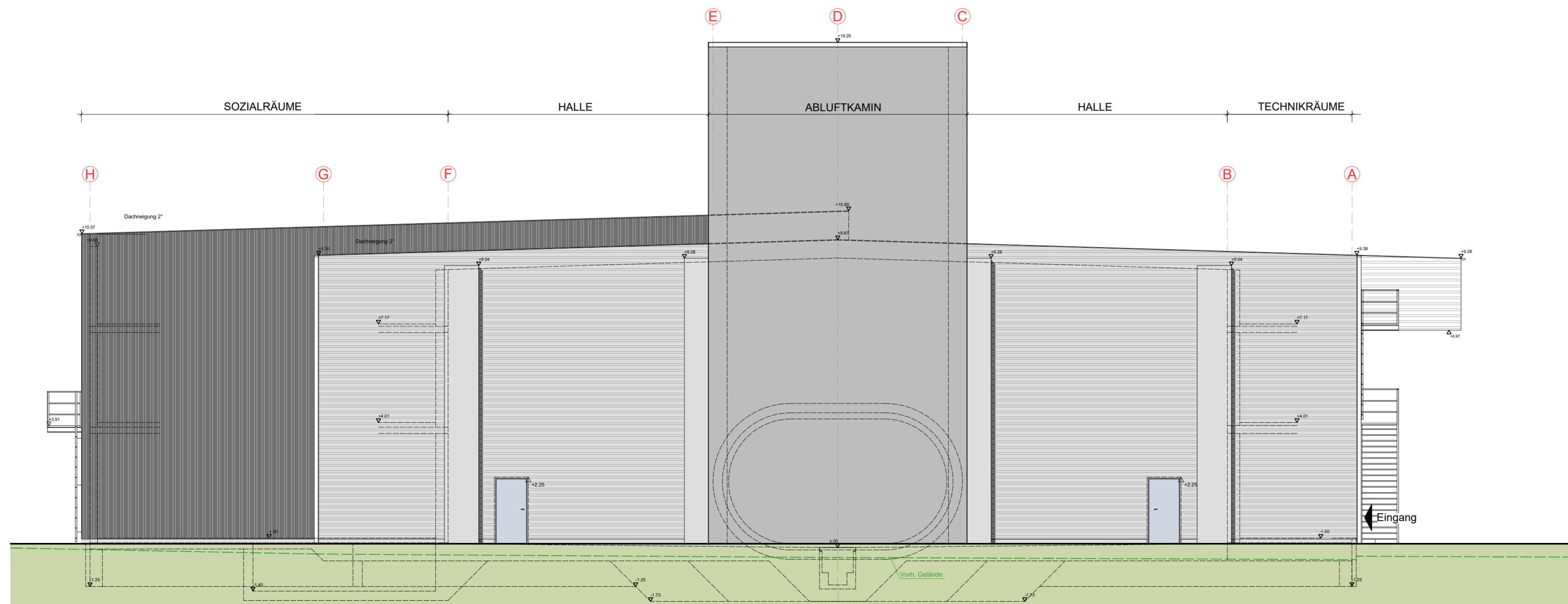
Nord-Ansicht
