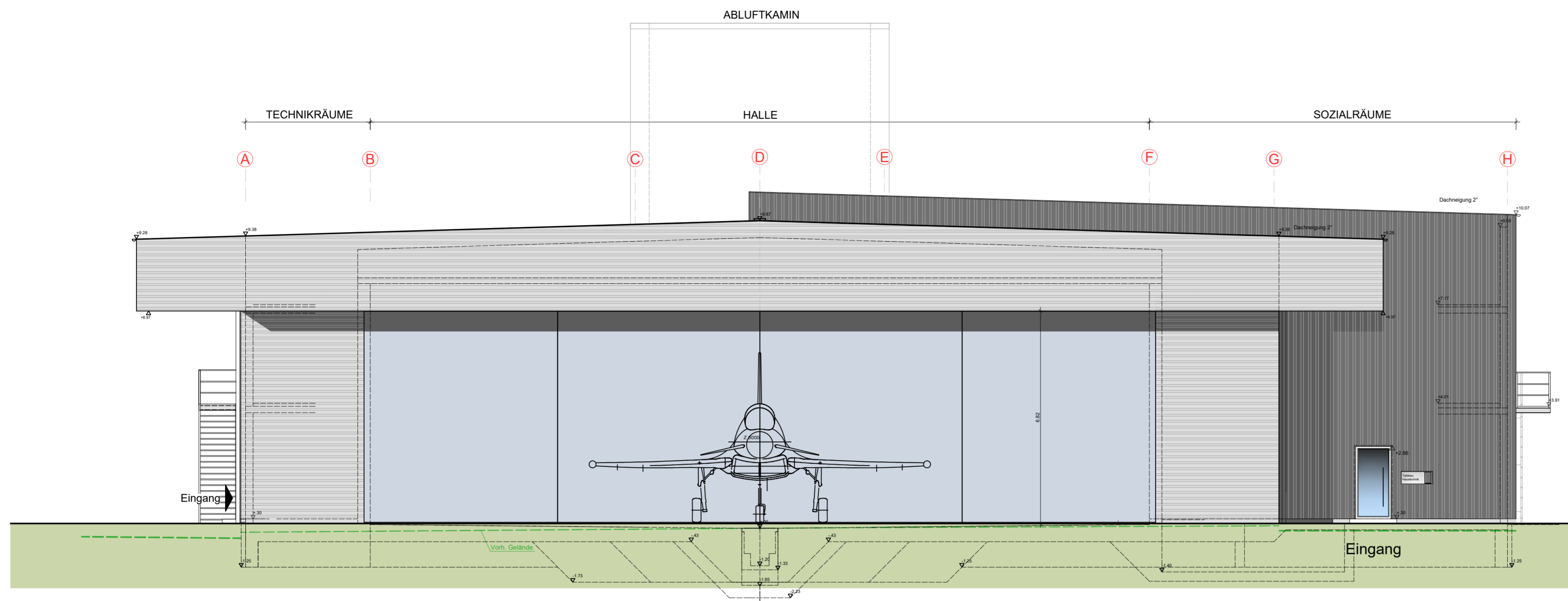
Süd-Ansicht
